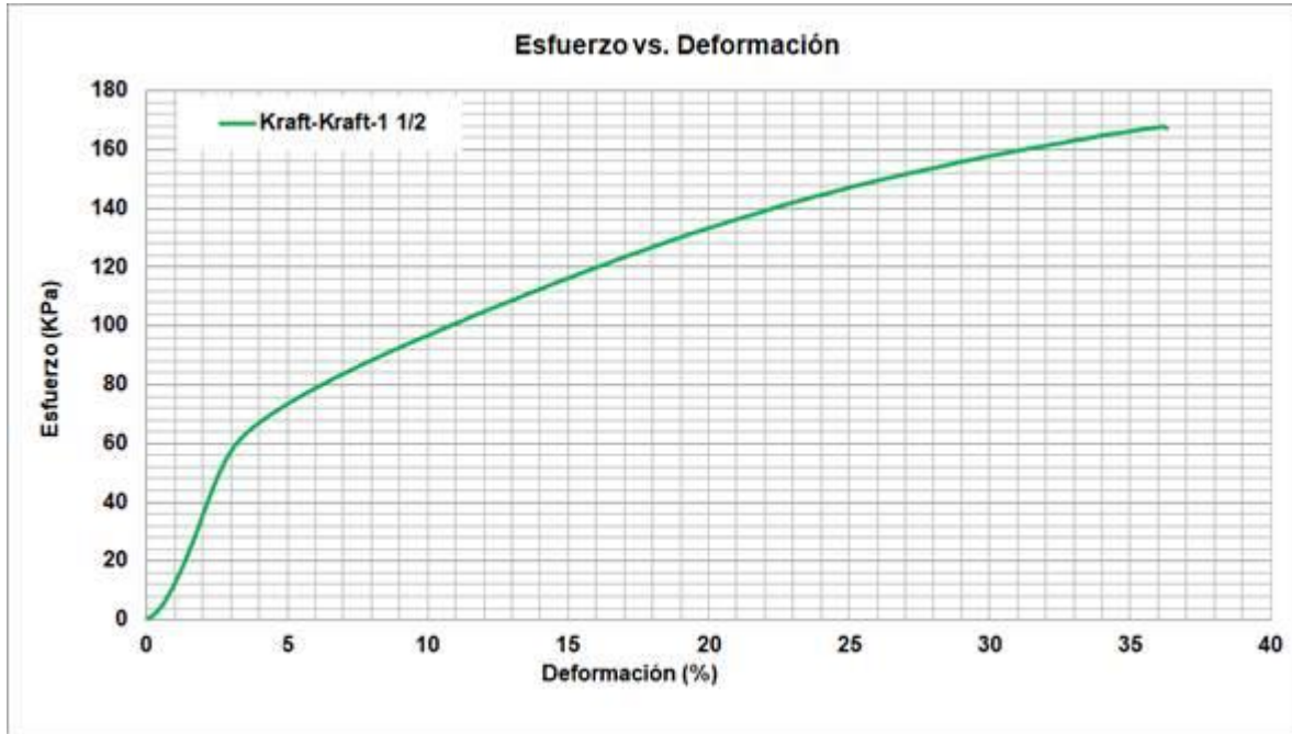
Figura 3. Curva de esfuerzo (KPa) vs. deformación (%) de la muestra de la placa de poliuretano Kraft/Kraft standing seam espesor 1 1/2 pulg.
