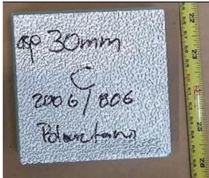
Figura 1. Probeta para el ensayo de compresión.
